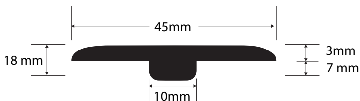
T-molding
