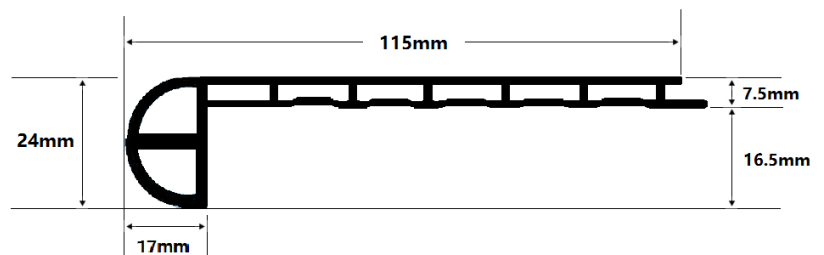
Flush stairnose
