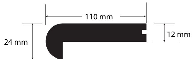
Flush Stairnose
